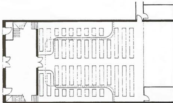
PLANTA A LA ITALIANA DEL TEATRO CALDERON
