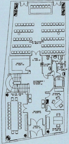
PLANTA BAJA
