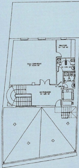
PLANTA ATICO
