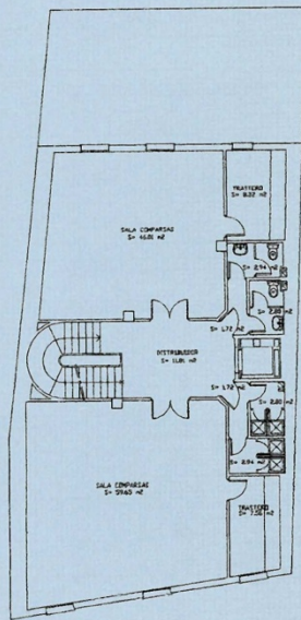
PLANTA SEGUNDA Y TERCERA
