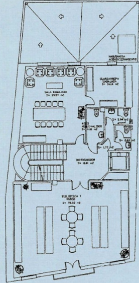
PLANTA PRIMERA
